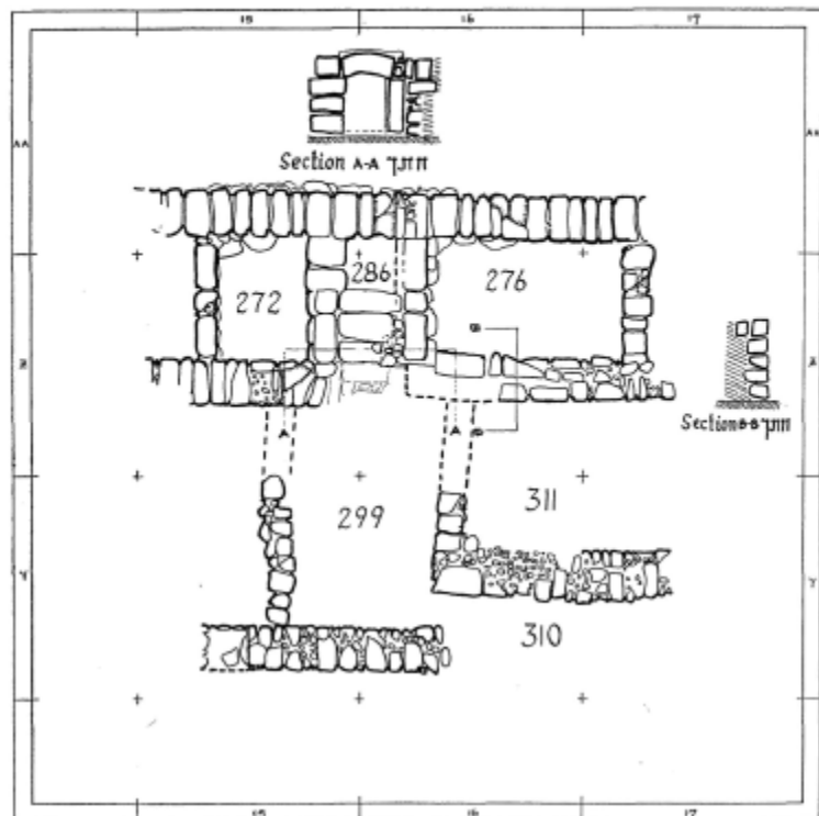
ציור 8. תכנית הקטע הצפוני של חומת הסוגרים ומעבר-הסתרים.
