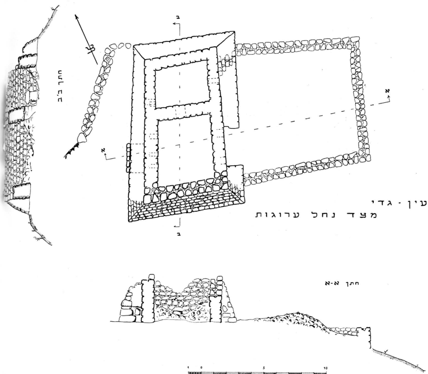
ציור 8. מצד נחל ערוגות (23).
