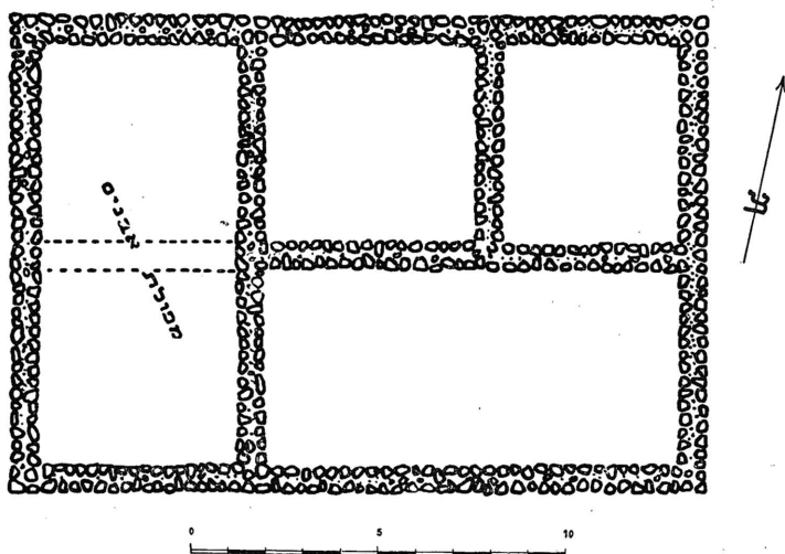
ציור 5. בנין מעל למצפה עין-גדי (6).
