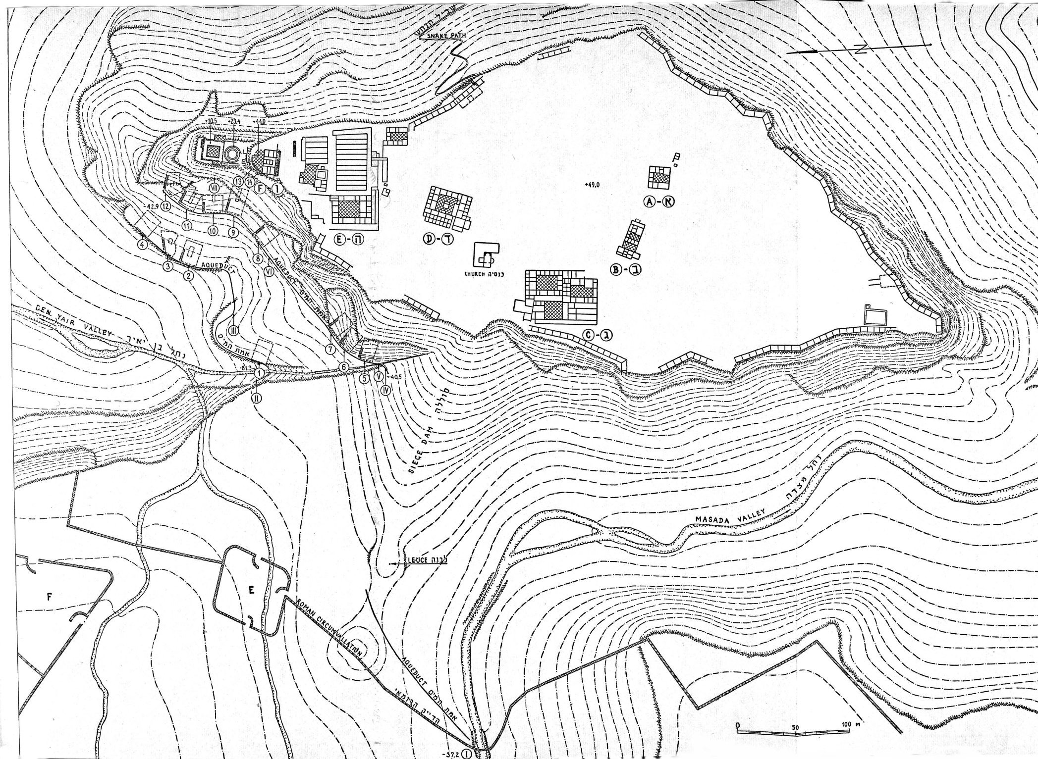
ציור 3. תכנית המבצר ומתקני המים שלו
