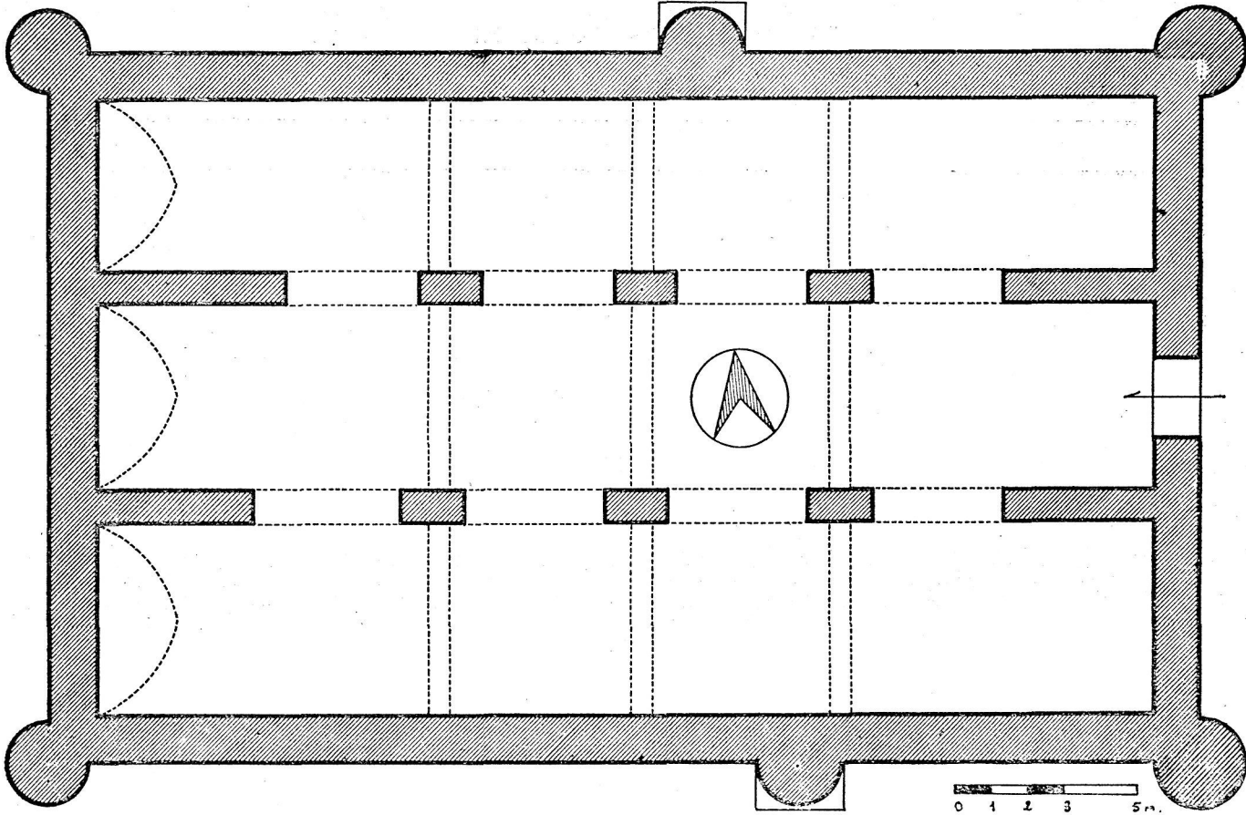
Şek. 3 - Tatvan Ham. Restitüsyon planı.
