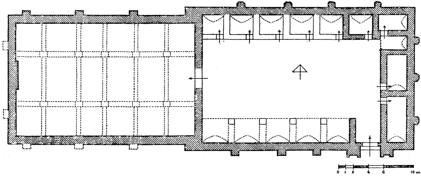
Şek. 5 - Çingene Hanı'nın, Sayın Celâl Yalvaç'ın aldığı ölçülere göre çizilmiş planı.
