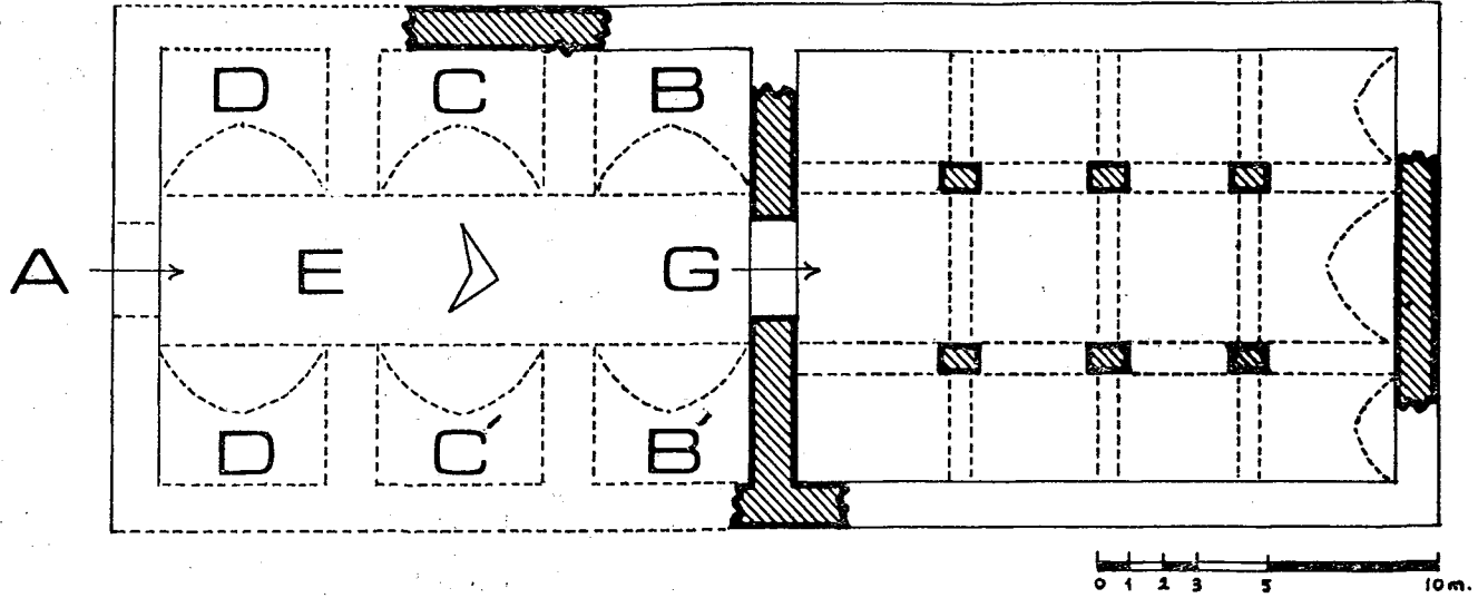
Şek. 1 - Kamereddin Hanı planı.
